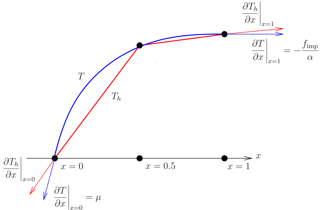
FIGURE 9.1: Problème de diffusion 1D à 3 points (9.17).
