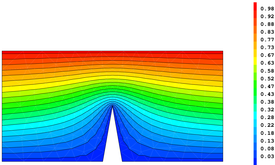
FIGURE 2.8: Isovaleurs de la solution discrète V_h du cas du paratonnerre.
