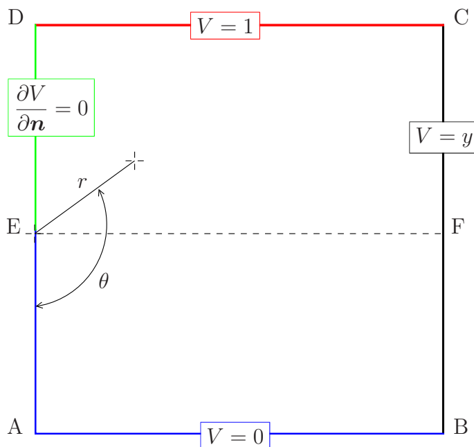
FIGURE 2.9: Schéma représentant un demi-domaine \Omega et les conditions aux limites associées au cas du paratonnerre, figure 2.7, lorsque \alpha = 0 .
